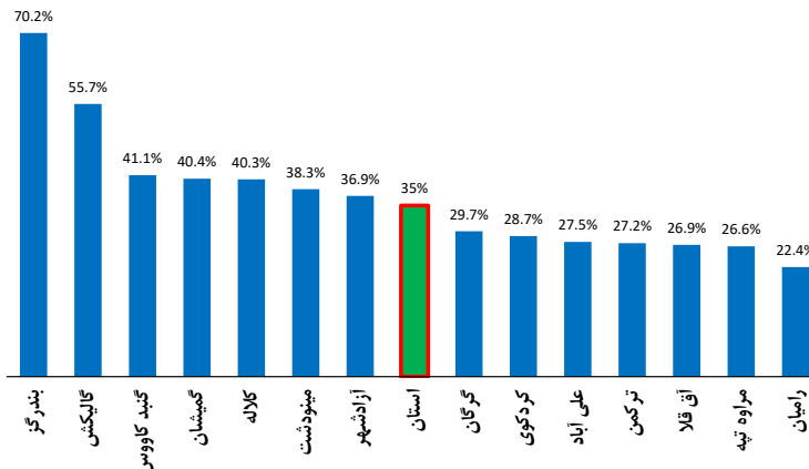
درصد تغییرات بارش تجمعی مهر لغایت آذر سال جاری نسبت به دوره درازمدت
